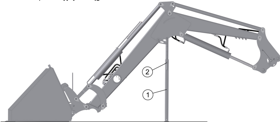
Rys. 8. Sposób ustawienia wysięgnika z narzędziem roboczym na podporach po wymontowaniu z przyłącza.
