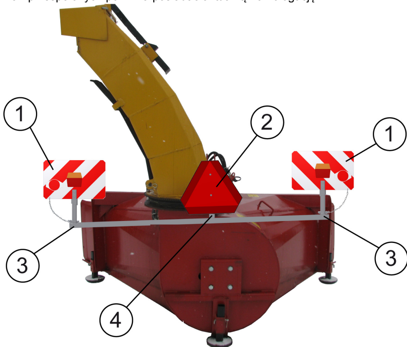
Rys. 3 Urządzenia świetlno-ostrzegawcze
